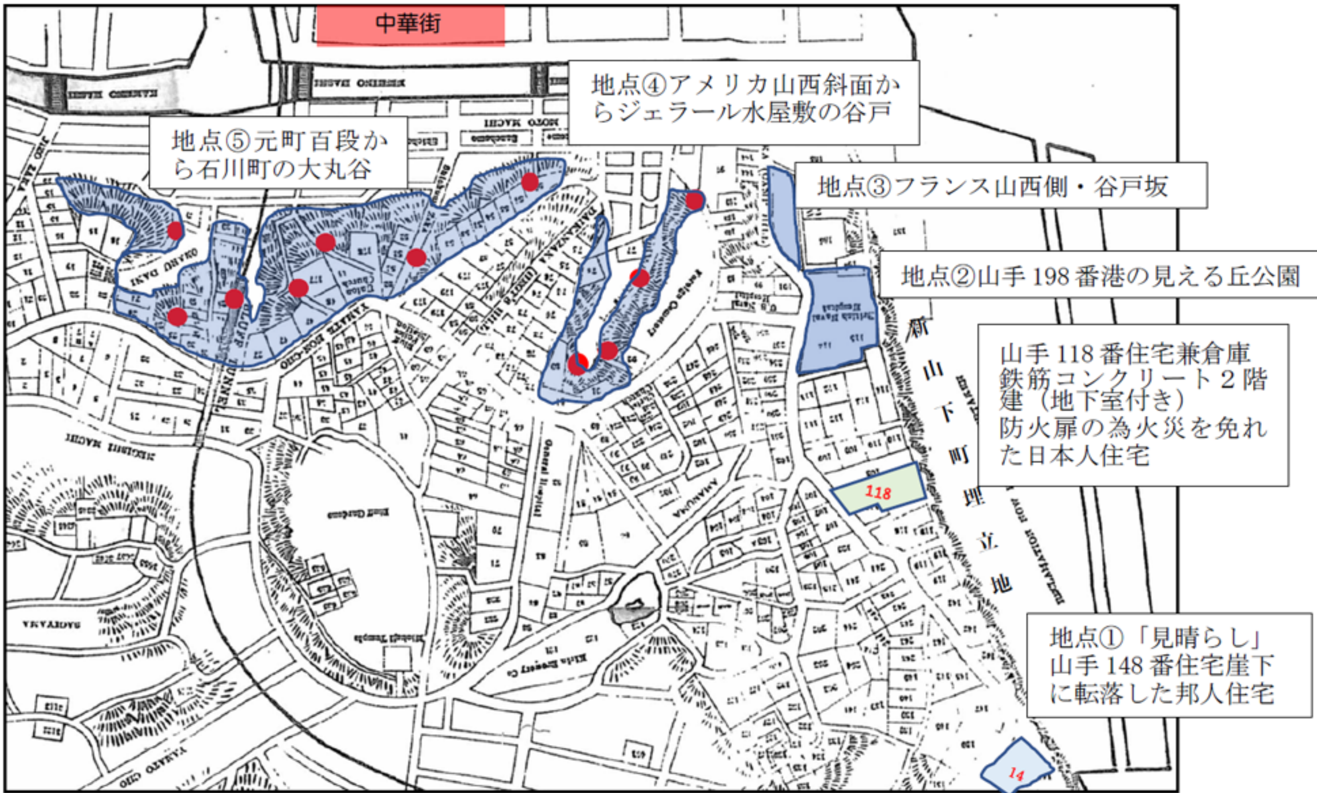
図5 本牧台地東部の被災地（BLUFF DIRECTORY, 1923）●は本文の記載場所の位置を示す
