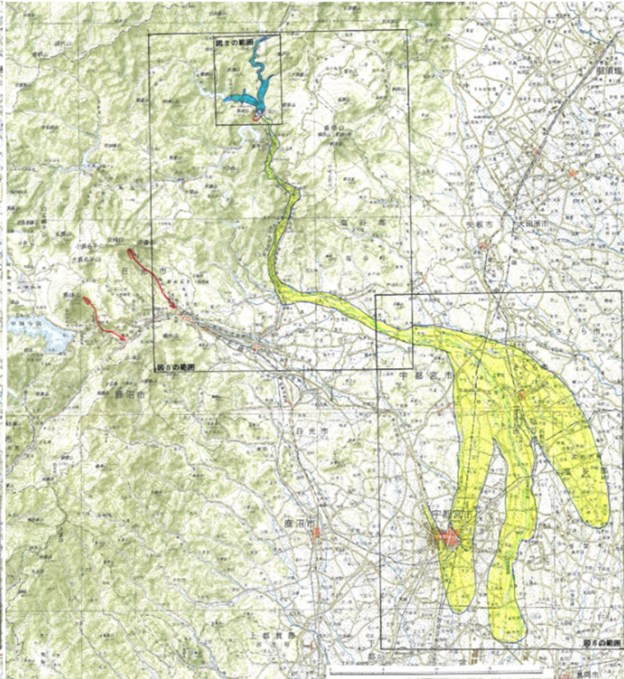
図3 1683年の葛老山の崩壊と天然ダム、40年後の決壊洪水の範囲 (越川, 1984をもとに1/20万地勢図日光・宇都宮・白川・水戸に追記)
