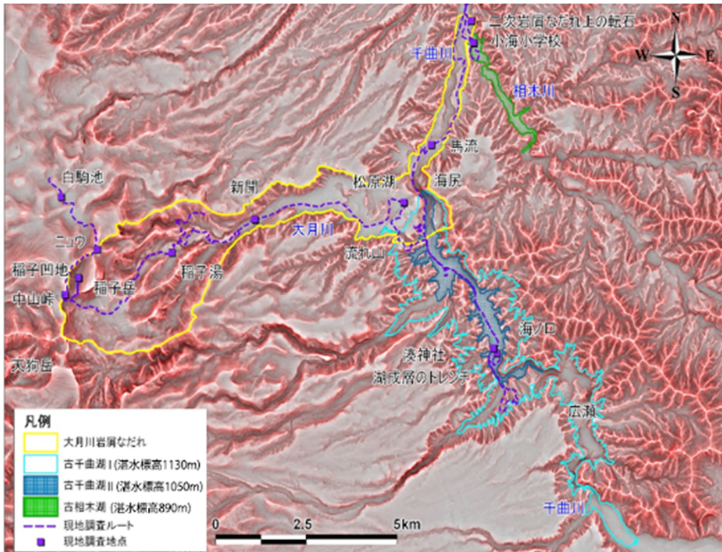
図2 千曲川上流部の大月川岩層なだれと天然ダム的位置 (井上ほか, 2010)
