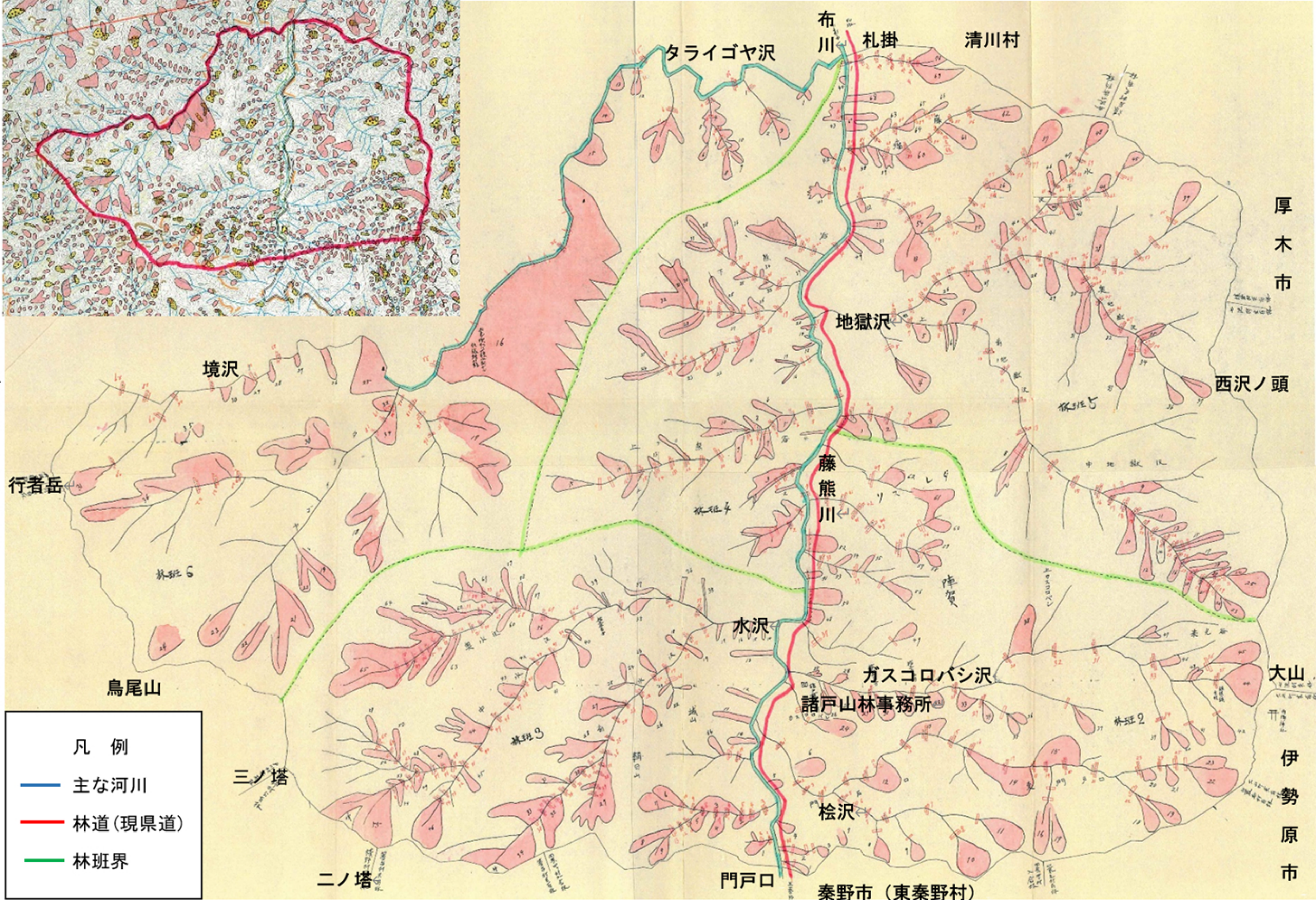
図5 諸戸山林の関東地震直後崩壊地分布図(勝沼(1924)『中津川流域荒廃地調査報告』の附図) 原図は東京大学砂防工学研究室(現 森林生物地球科学研究所所蔵) 左上図は諸戸山林地域の自然災害履歴図(コラム93の図4参照)
