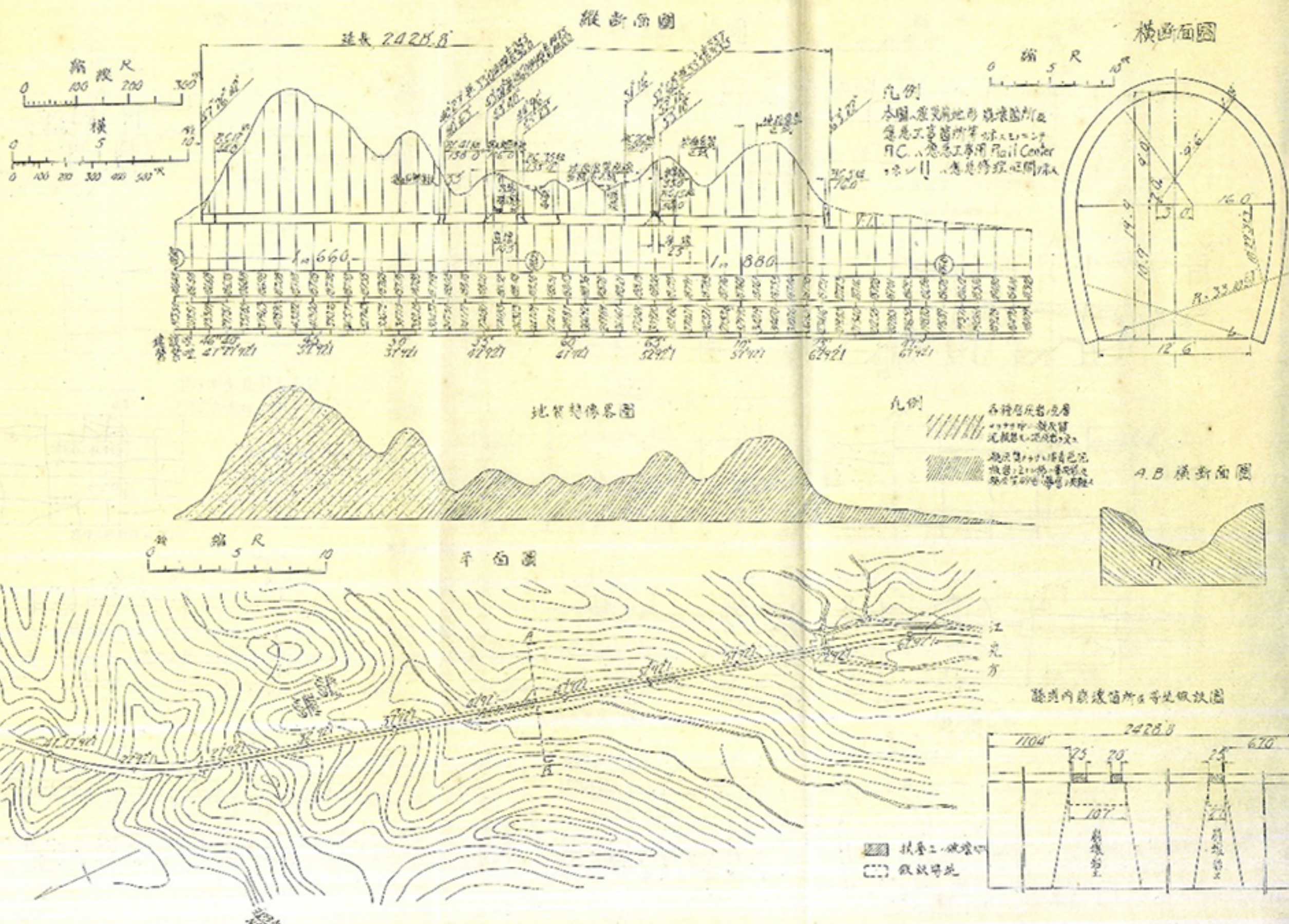
図6 國有鐵道北條線南無谷隧道全般圖（附圖第九十三）（復興局，1926）
