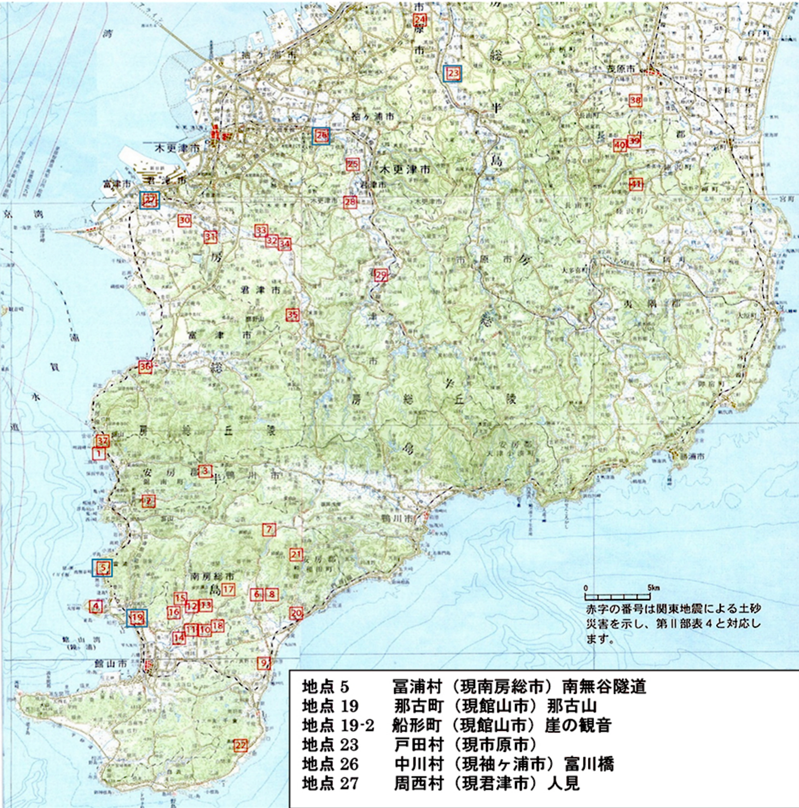
図3 関東大震災による千葉県南部の土砂災害分布図（井上編著，2013）
