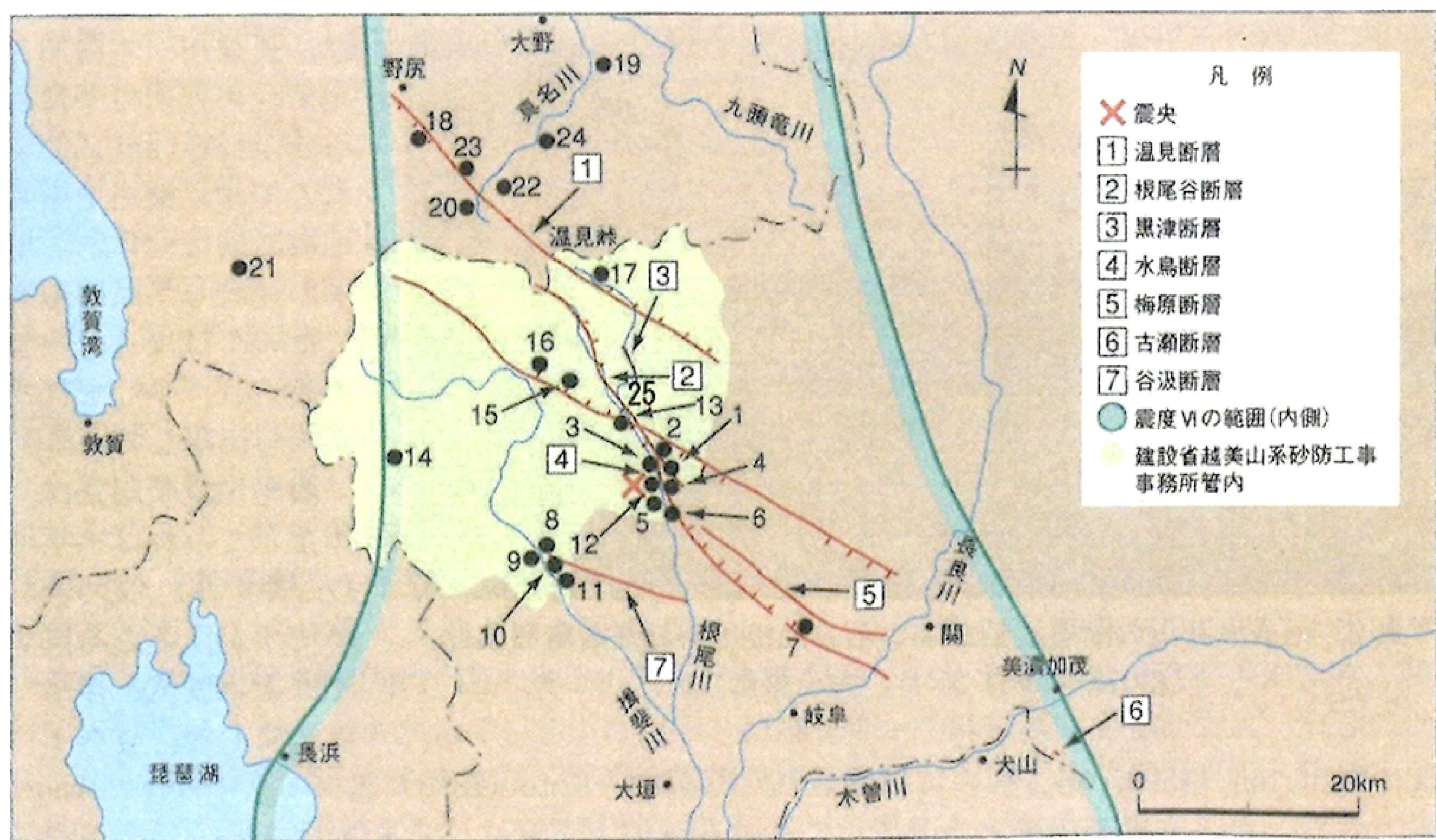
図5 濃尾地震に関連した地震断層・土砂災害等の一覧図
