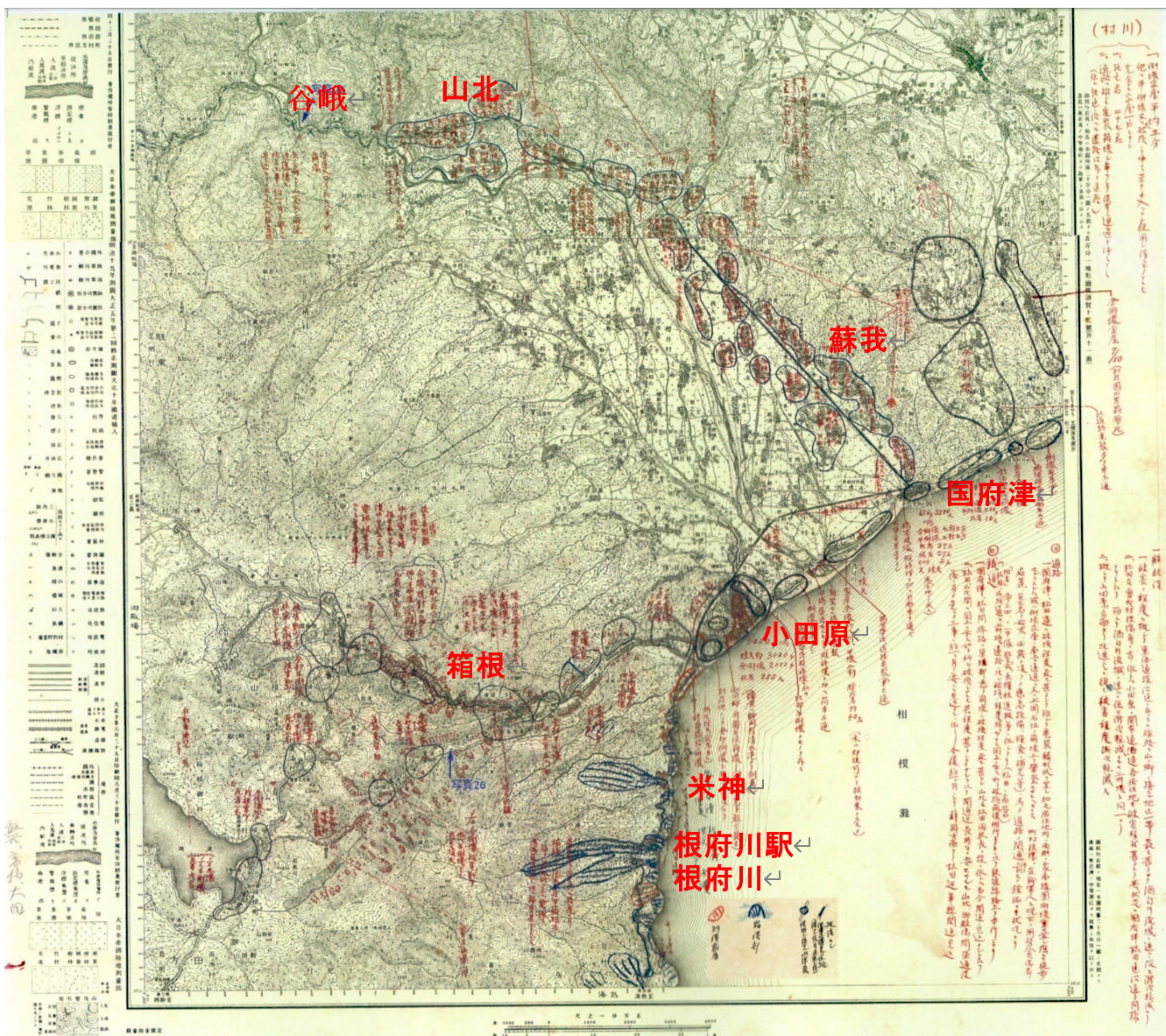
図2 震災地応急測図 1/5 万地形図「小田原「松田総領」図幅」 (歴史地震研究会編集, 2008; 井上編著, 2013; 井上, 2017)
