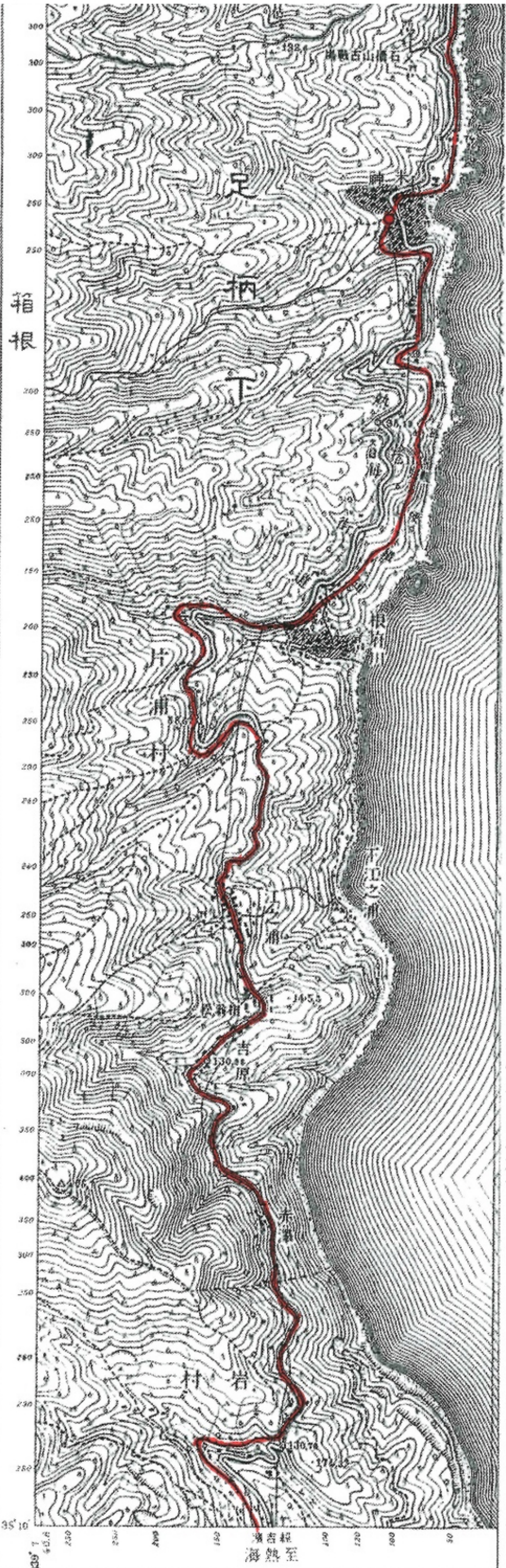
図1 1/2.5万旧版地形図「小田原」図幅（左：1916年修正、右：1933年修正） （関東地震前後の小田原市石橋～江ノ浦間の地形と土地利用の比較）
