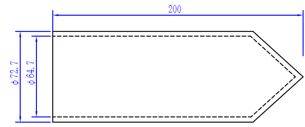
パイロットキャップ 4型 S=1/3 φ72.7/64.7×200
