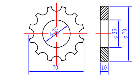
スペーサー 2型 S=1/3 φ70×10
