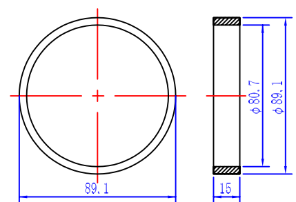
スチールリング4型 S=1/3 φ89.1×15
