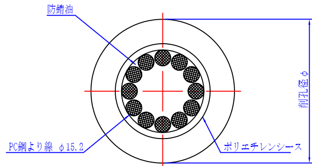
A-A断面図 S=1/3
