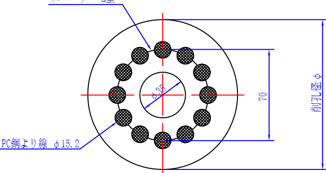
B-B断面図 S=1/3
