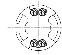
A-A断面
